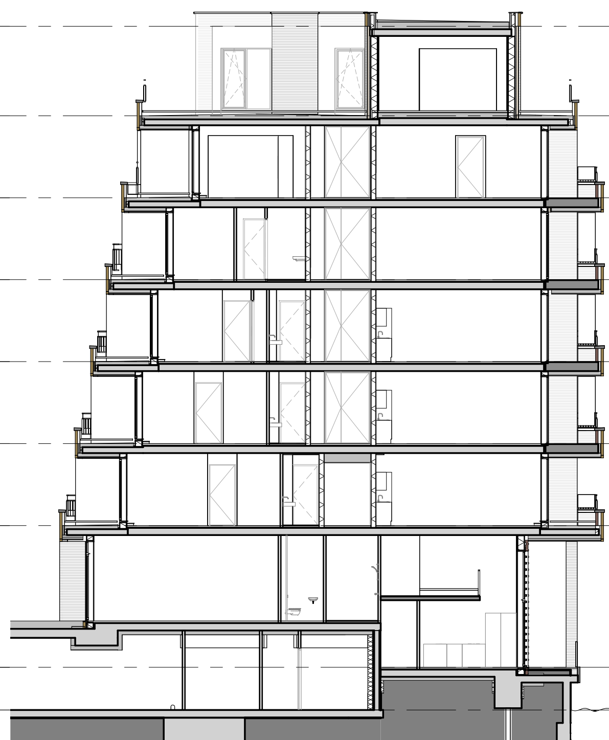
Doorsnede B-B - Oost beuk
