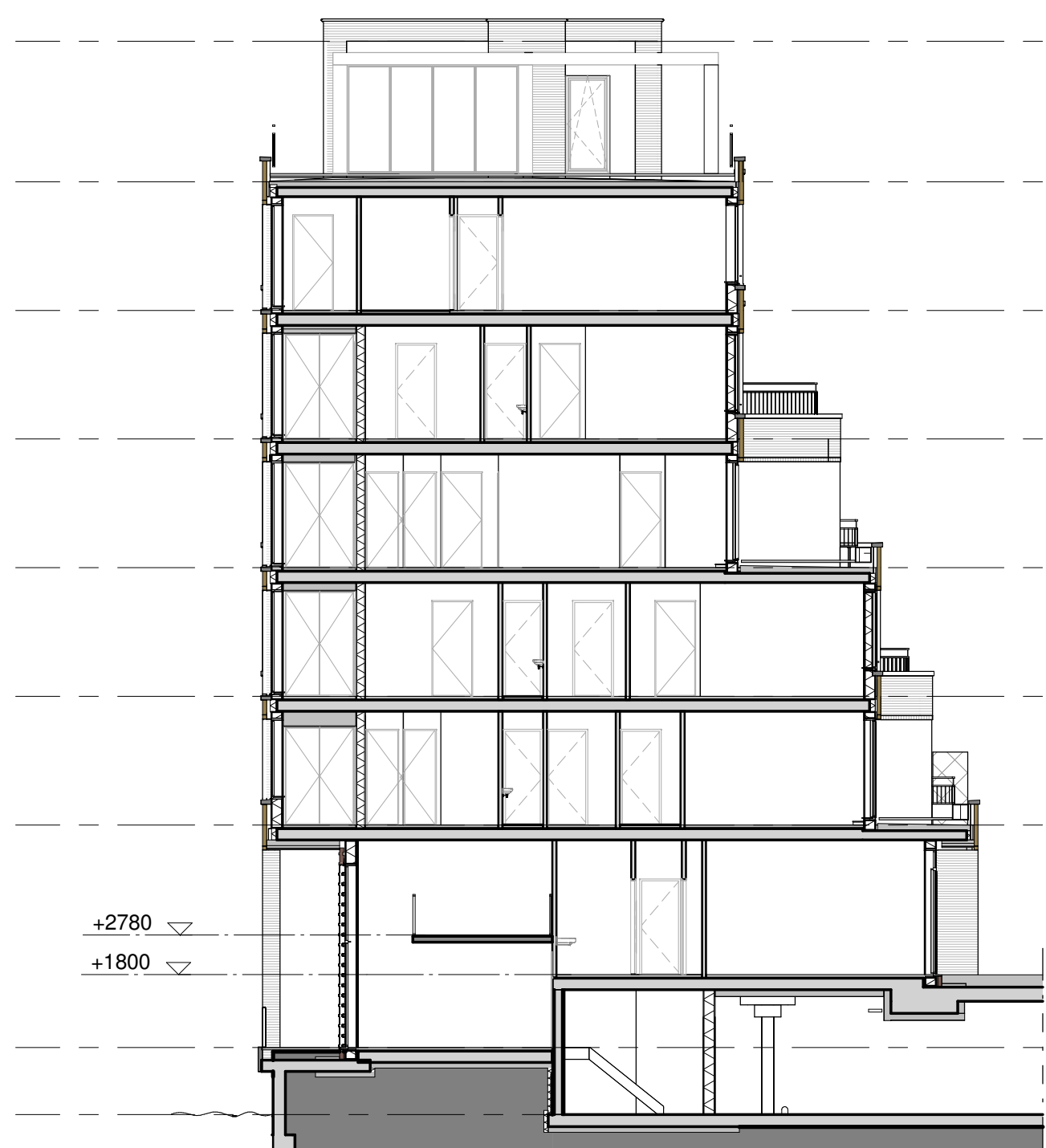
Doorsnede A-A - Noord beuk
